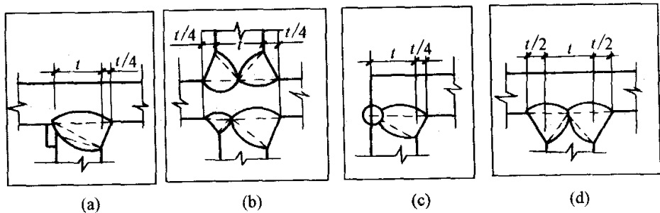
图 5.2.5 焊脚尺寸
